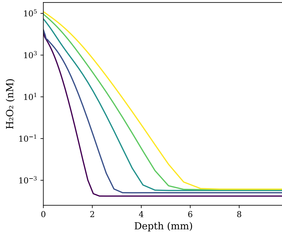
(d) \text{H}_2\text{O}_2
